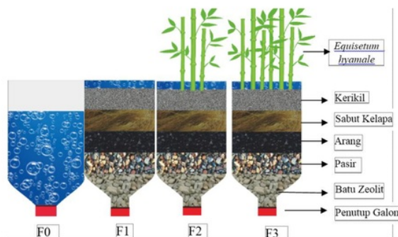
Gambar 1. Desain Reaktor
